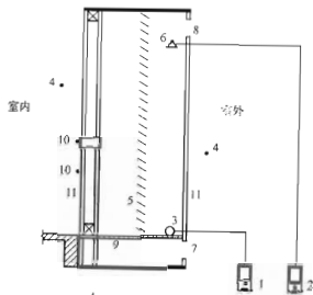
图1 双层幕墙热通道通风量检测系统
