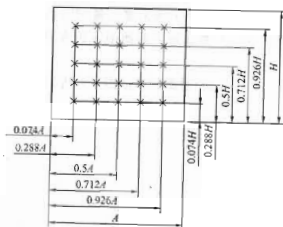
图 E.1.3-1 矩形风管 25 个测点时的测点布置
