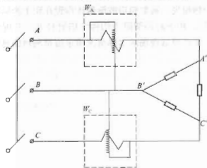
图 2 两表法测量电机输入功率原理
